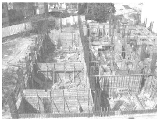
4 10/20教學大樓地下室B1F內牆及1FL樓版及樑模板組立施工照片
