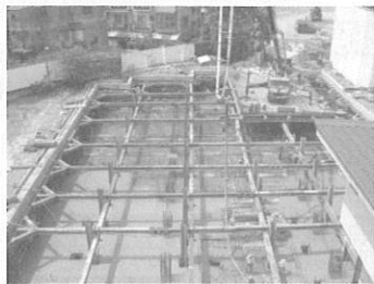
3 9/29教學大樓地下室筏基頂版澆置混凝土施工照片
