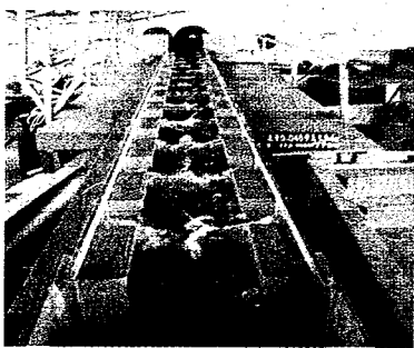
興大與水利署團打造創新「魚骨型魚道」，可幫助小型魚蝦順利洄游上溯。圖／王順昌提供
