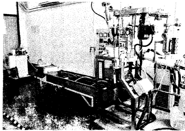
南臺科大購入10公升高壓聚酯反應器加造粒機等設備，全力支持產學共構技研中心運作。 南臺科大 / 提供
